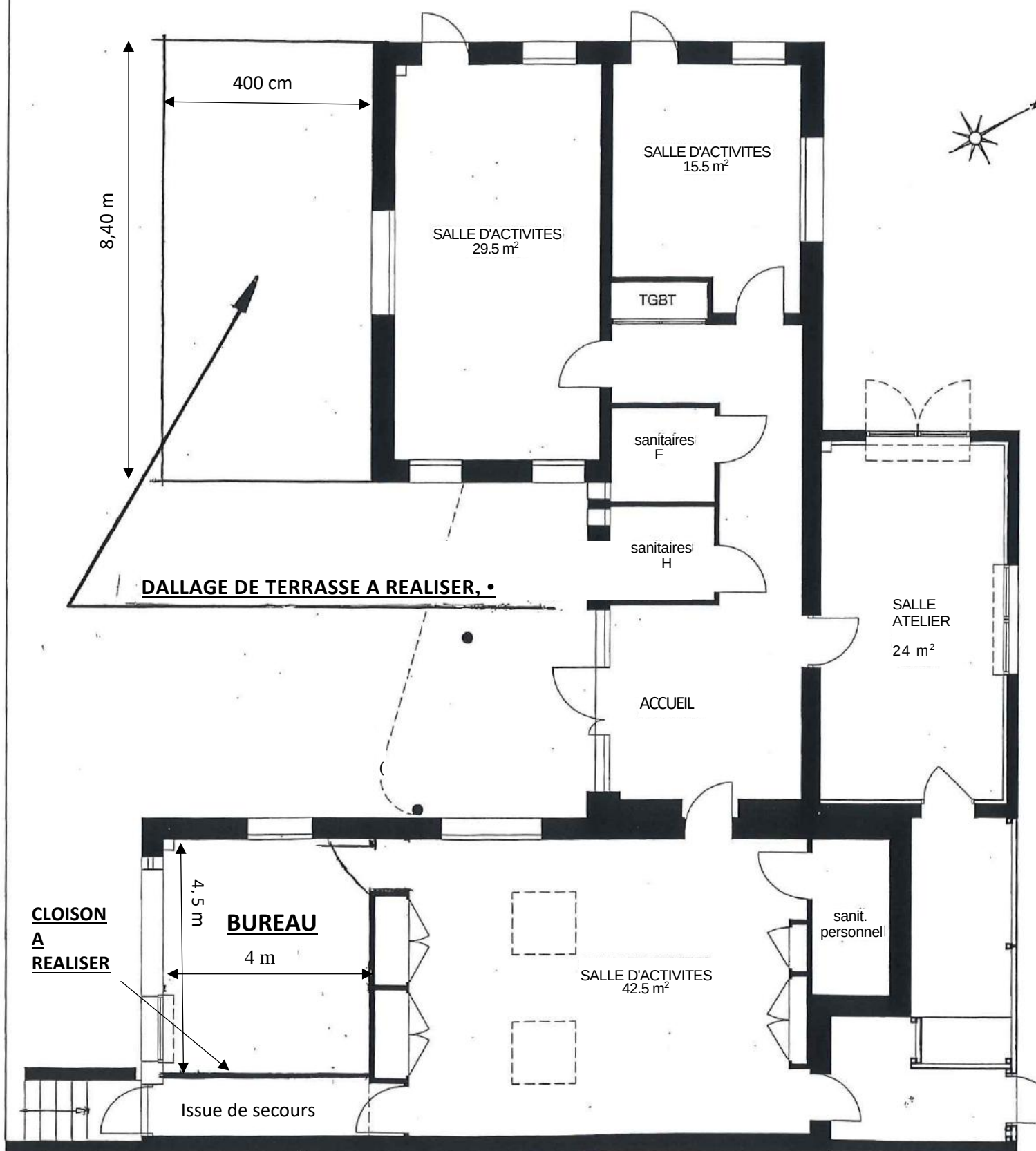
PLAN D'ENSEMBLE DU LOCAL - ETAT EXISTANT
